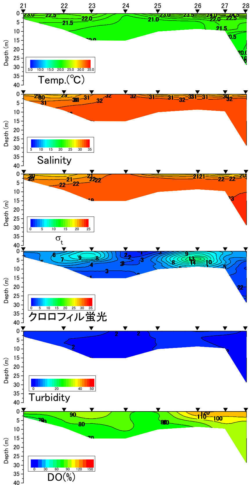
有明海東ラインの水温(°C)、塩分、密度( \sigma_t )、クロロフィル蛍光強度、濁度、溶存酸素飽和度(DO%)の鉛直面図(国土交通省の調査による) (2016年6月14日)
